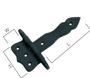
3790 MB L90xW39xH58mm
